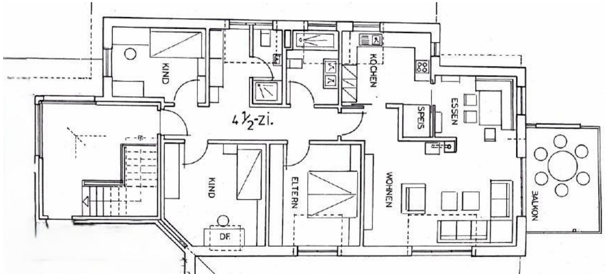
Dachgeschoss
