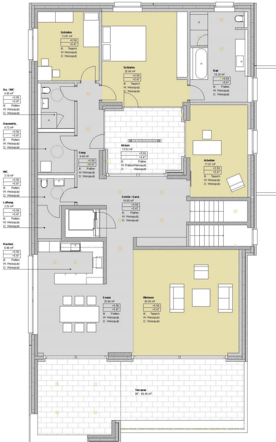
Wohnung Obergeschoss 187.82 m 2 Mst. 1:100
