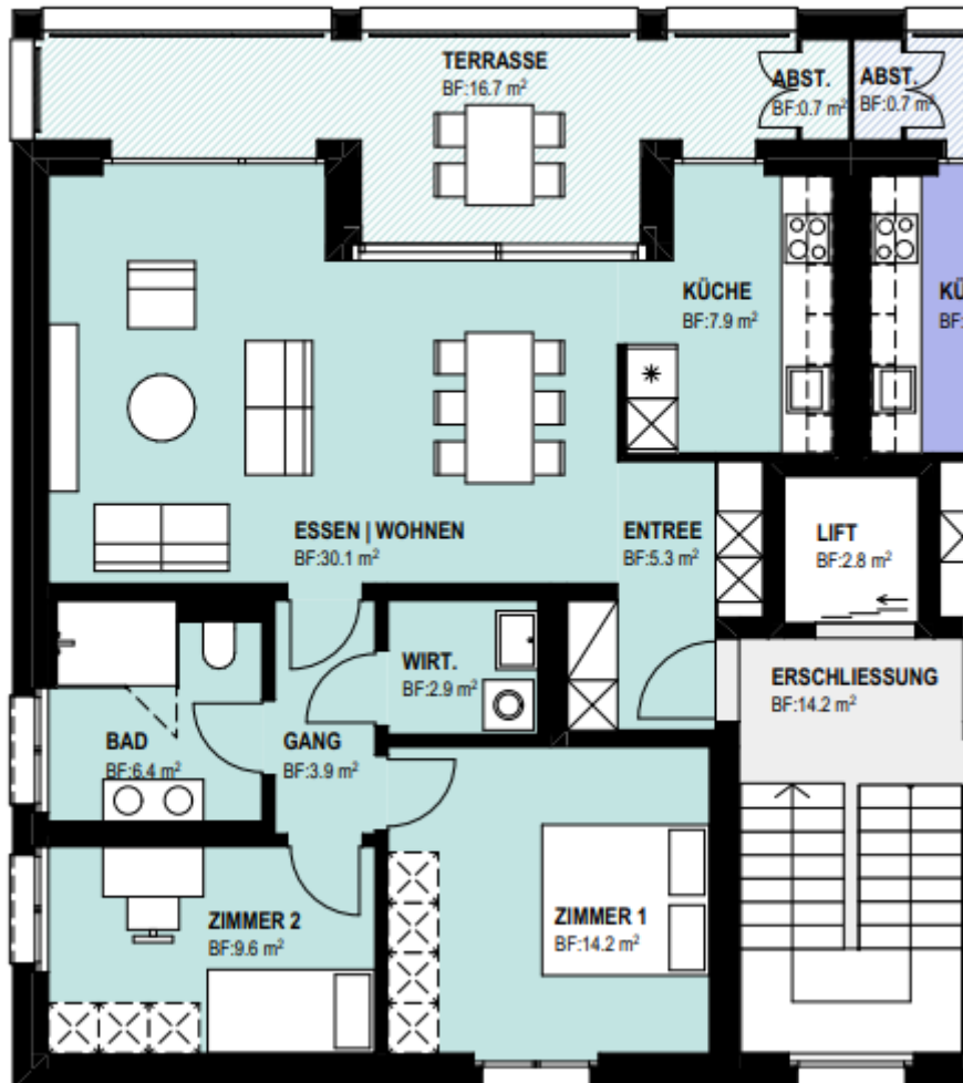
Attika Wohnung Süd-Ost
