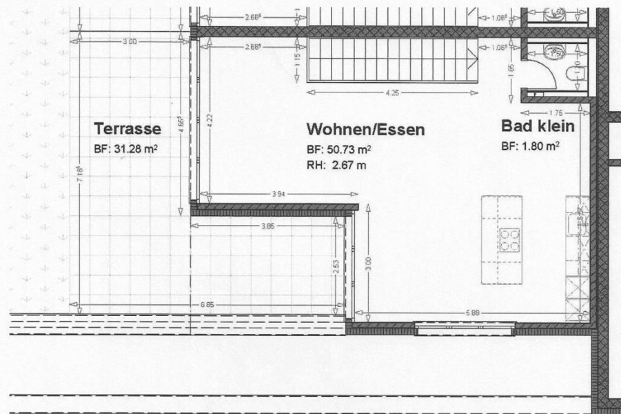
Grundriss Ebene 6
