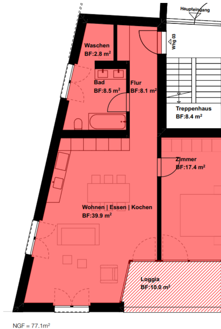
Erdgeschoss
