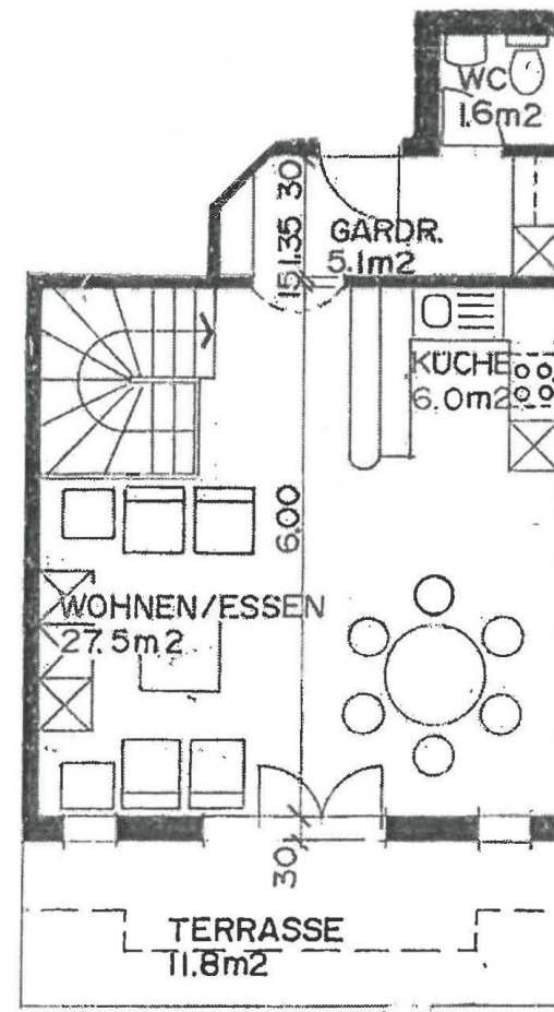
1. OBERGESCHOSS 1:100
