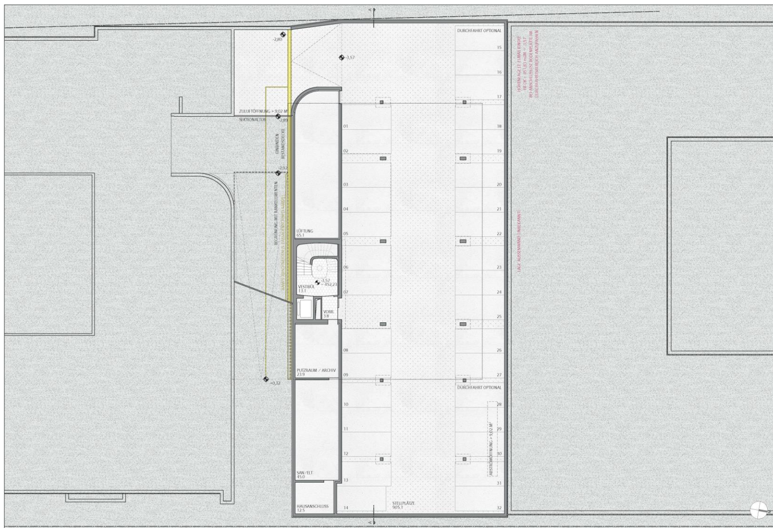
Untergeschoss
