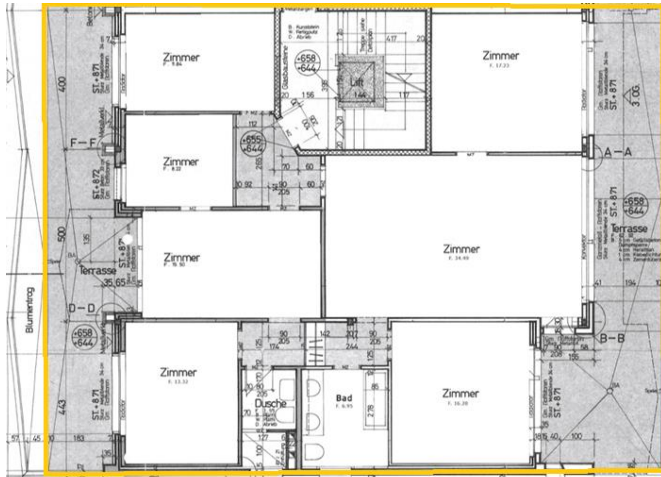
2. Obergeschoss
