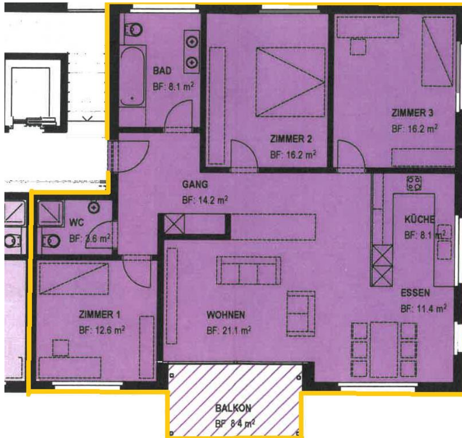
2. Obergeschoss
