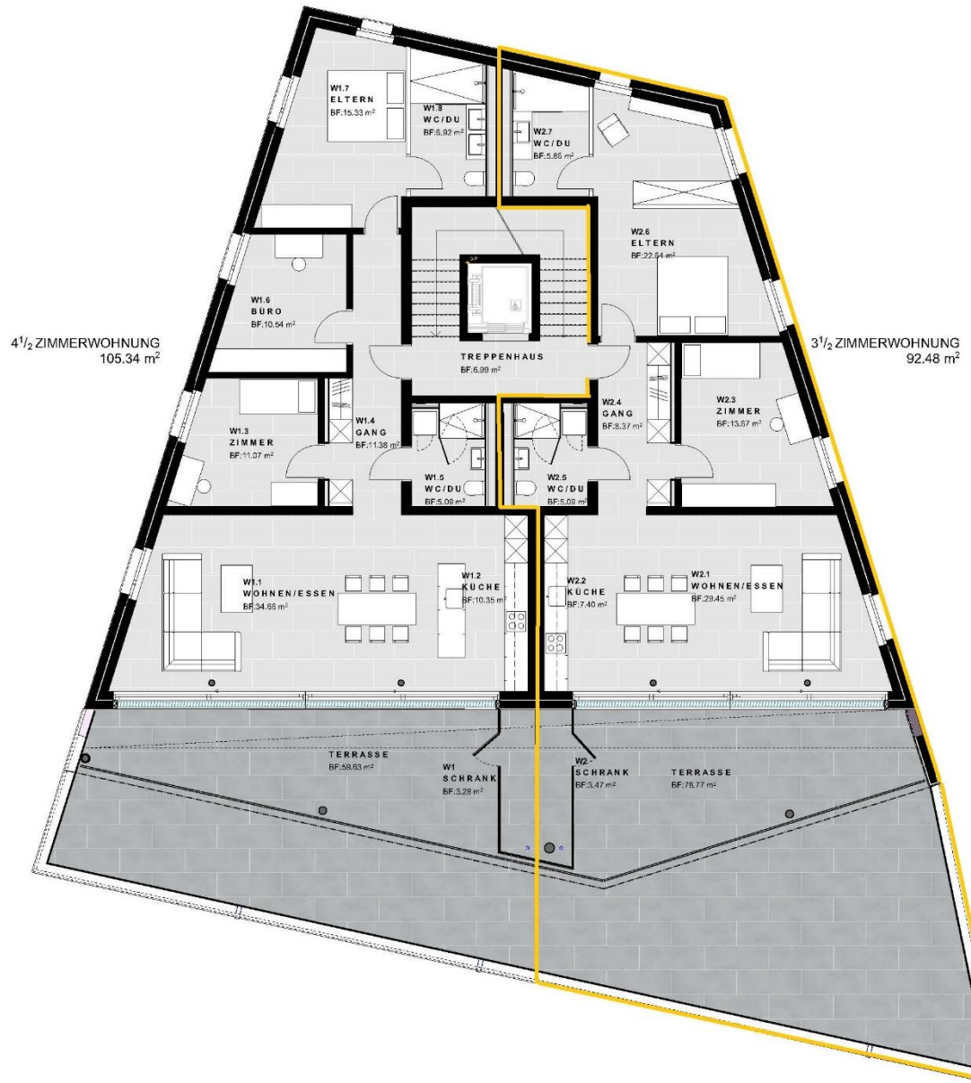
3.5 Zimmer-Wohnung EG
