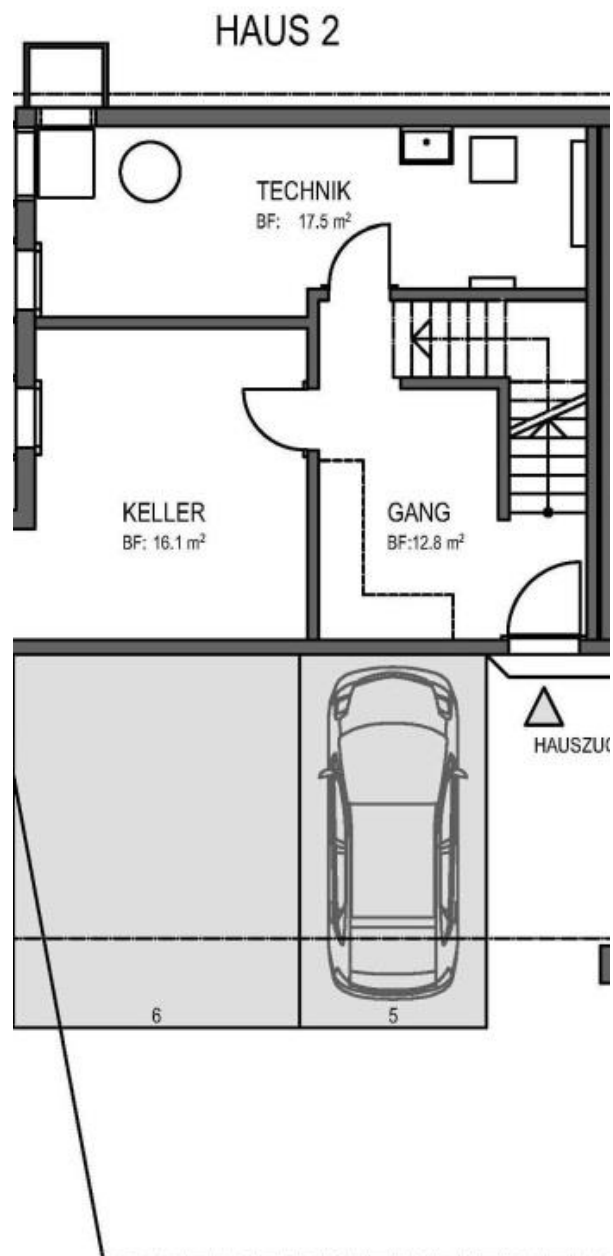
Grundrissplan Untergeschoss
