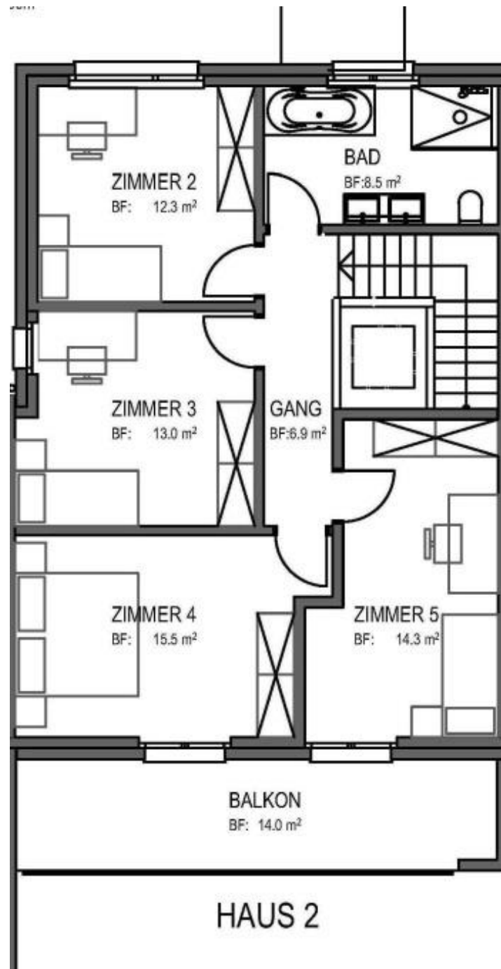
Grundrissplan Obergeschoss
