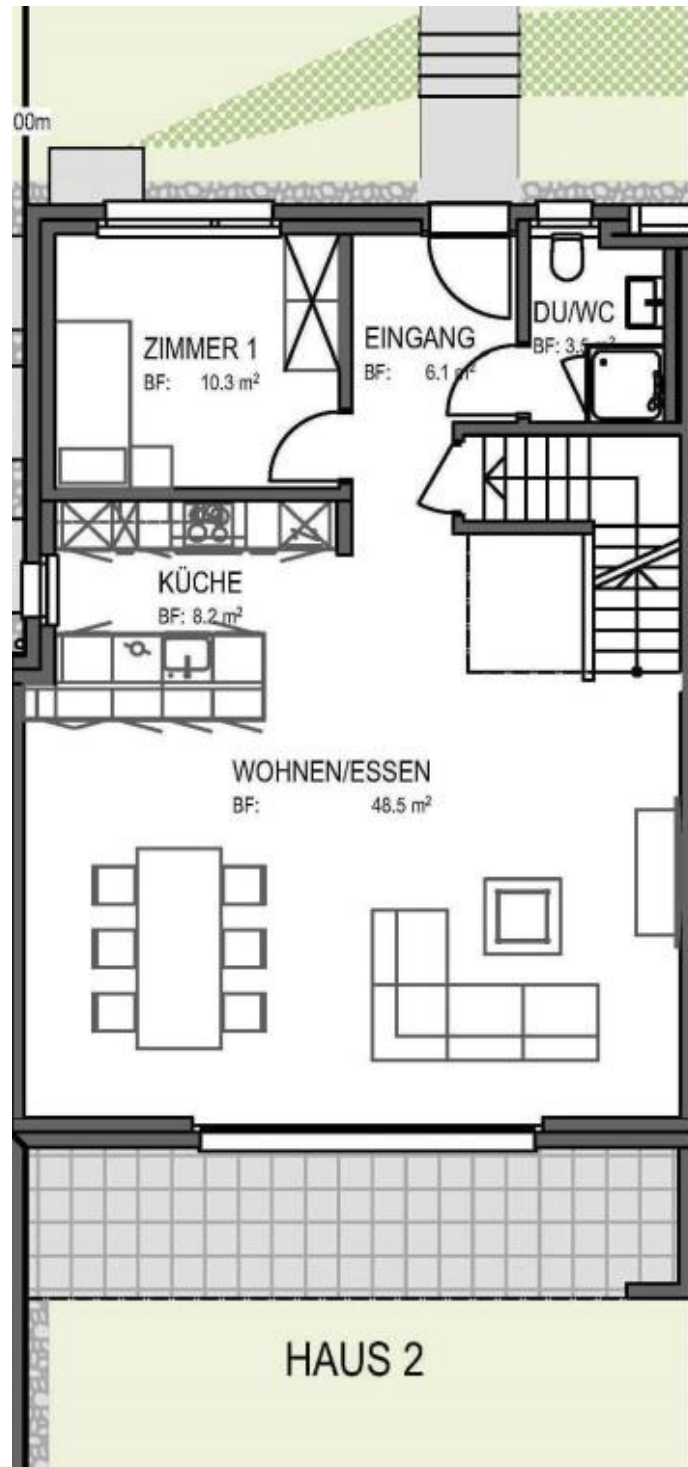
Grundrissplan Erdgeschoss
