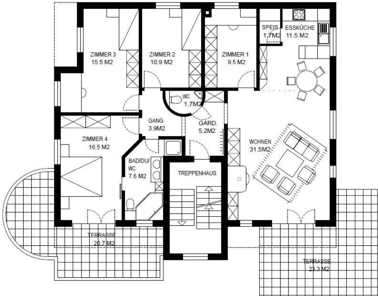
1.OBERGESCHOSS M 1/100 Wohnung 7
