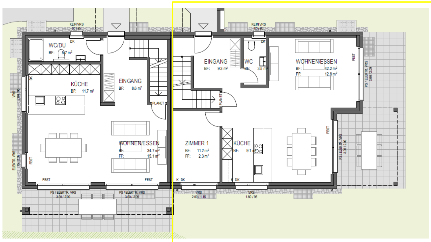
Erdgeschoss
