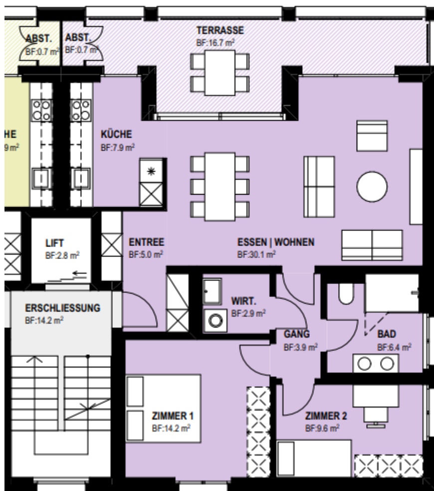
2.Obergeschoss Wohnung Süd-West
